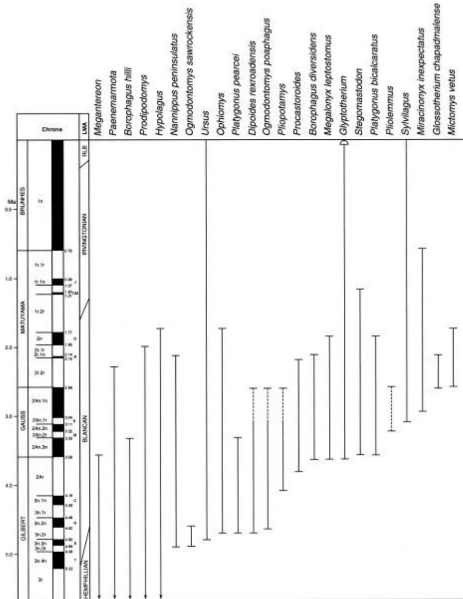
Figura 3. Rangos temporales de algunos mamíferos de América del Norte del Plioceno y Pleistoceno. Las líneas punteadas indican un grado alto de incertidumbre.
