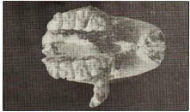
5) Merlionyx sewardi (órden de roedores) Eoceno, Mérid, Quauaquero.
