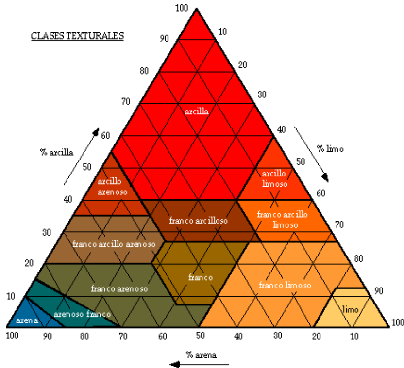
Figura 2. Clases texturales
