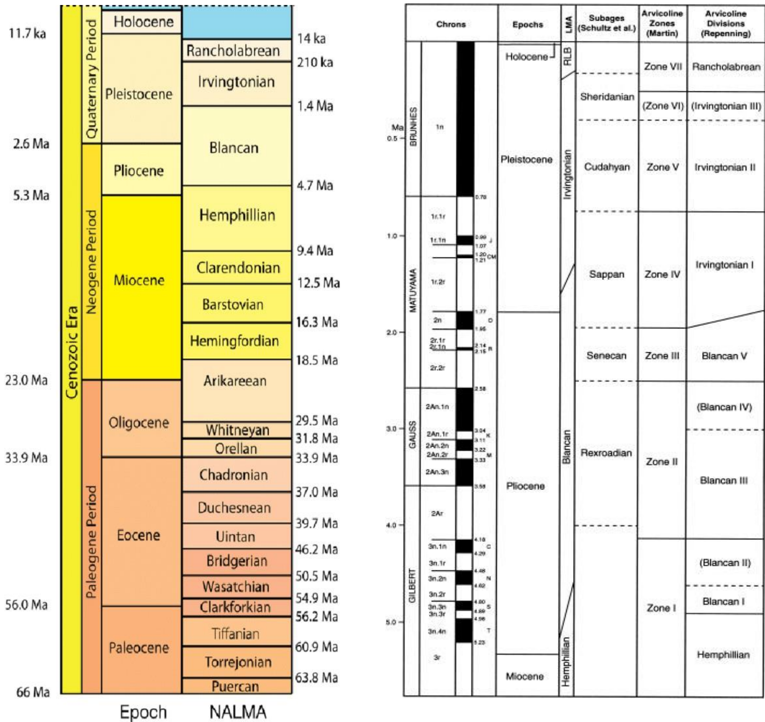
Figura 2. Izquierda división entre NALMAs (North American Land Mammal Ages por sus siglas en inglés o Edades de Mamíferos Terrestre de América del Norte). Derecha NALMAs de acuerdo con las divisiones cronológicas de roedores arvicolinos propuesta por Reppening y Martin (Tomado de Bell et al. 2004).
