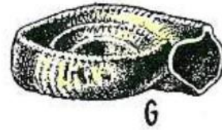
Eomphalus catillus Carbonífero. Inf.
