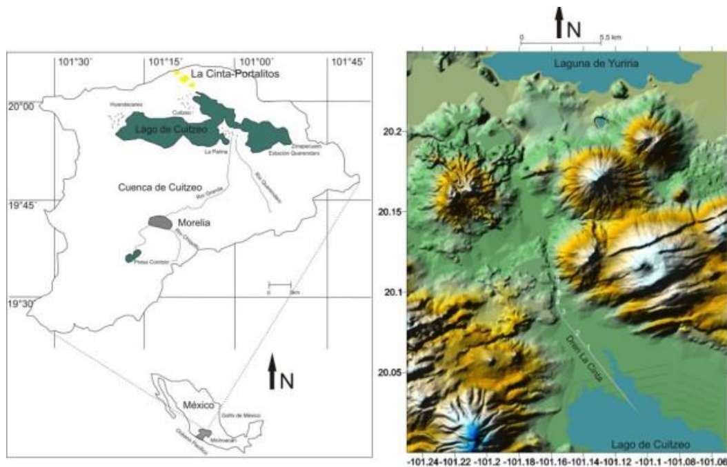
Figura 1. Ubicación de cuenca de Cuitzeo, Michoacán y Guanajuato (Tomado de Marín-Leyva 2011).
