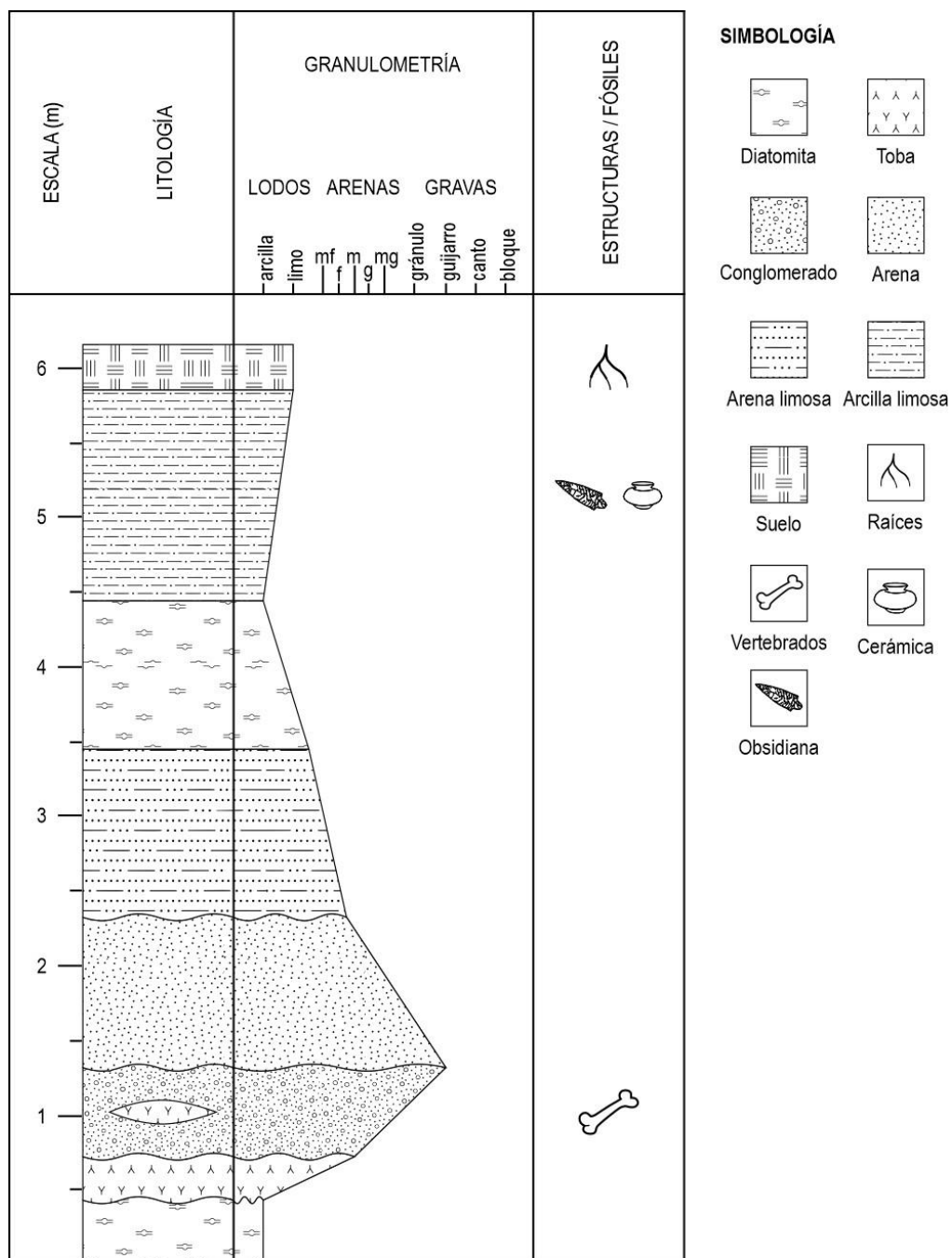
Ejemplo de columna estratigráfica individual, correspondiente a La Piedad-Santa Ana, una localidad el Pleistoceno tardío.
