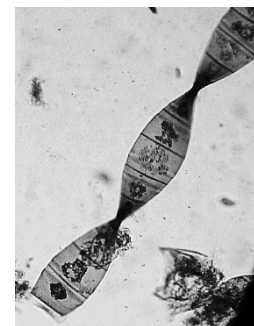
Helicotheca sp. (foraminífero)
