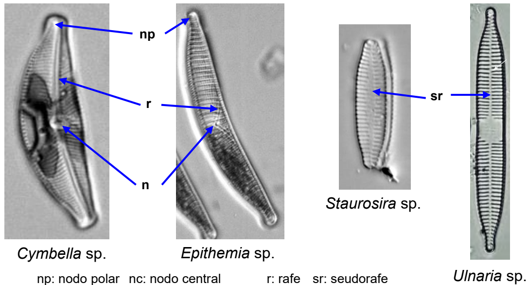
Figura 111. Rafe y pseudorafe.
