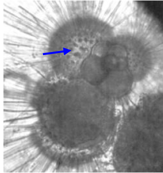
Globigerina sp. (Foraminífero con poros)
