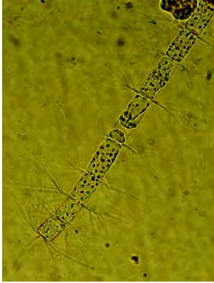
Bacteriastrum hyalinum Filamento simple recto
