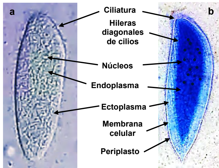
Figura 93. Opalina ranarum , trofozoito multinucleado, a) ejemplar vivo, b) ejemplar con tinción de azul de metileno)
