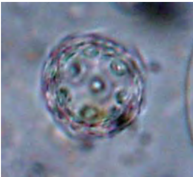
Umbilicosphaera sp. (cocolitofórido)
