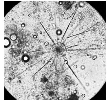
Acanthometron sp. (Heliozoario)
