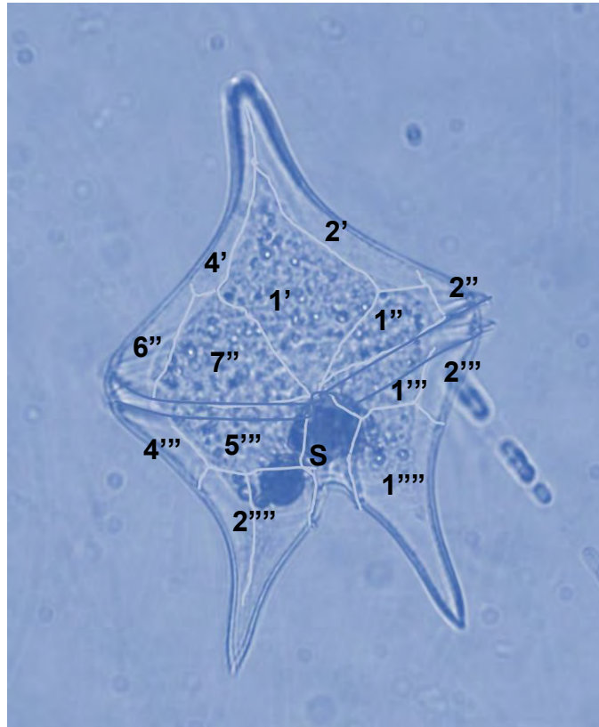
Disposición de las placas en Protoperidinium oceanicum .
