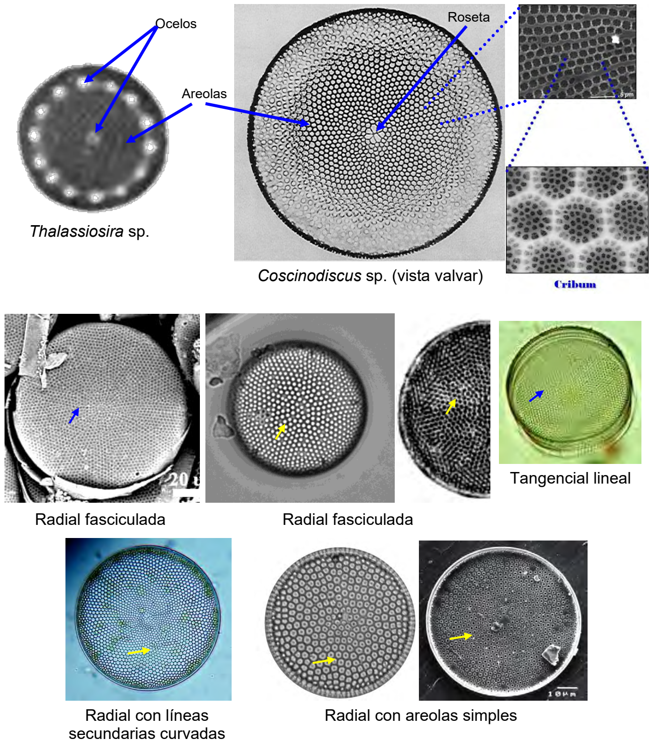
Figura 103. Diatomeas radiales con ocelos, areolas y crium
