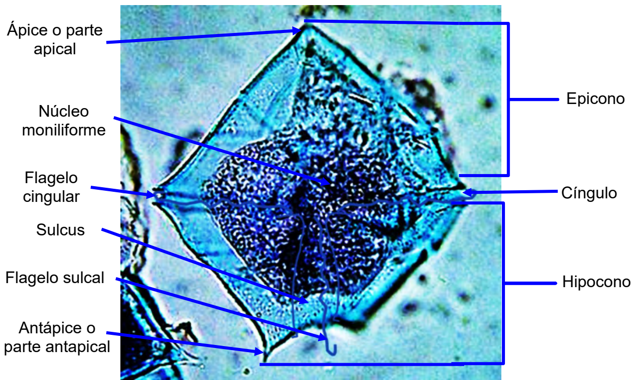
Figura 73. Principales estructuras morfológicas de un dinoflagelado tecado ( Protoperidinium sp.)
