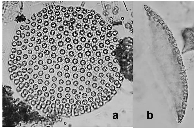
Figura 8. Talofita cenobial, Planktoniella muriformis (diatomea radial), cenobio en placa: a) vista de frontal, b) vista lateral.
