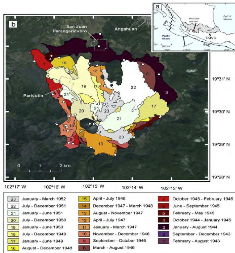
Fig. 4. Fases eruptivas del volcán Parícutin (Tomado de Larrea et al. 2017).
