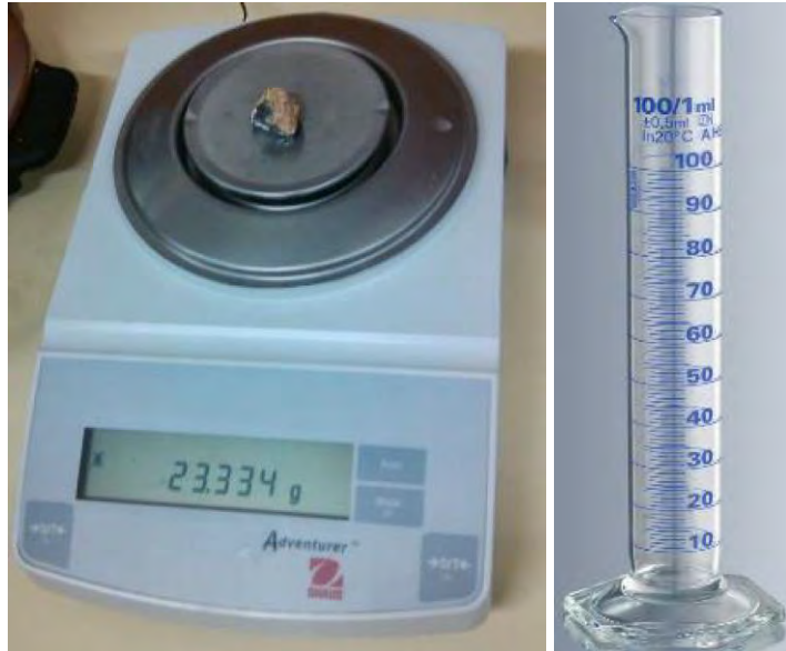
Figura 1. Balanza granataria y probeta graduada para densidad de las rocas.
